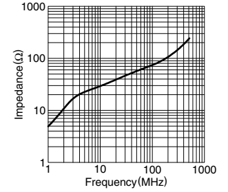
HF56SH18.8X1.1X15
